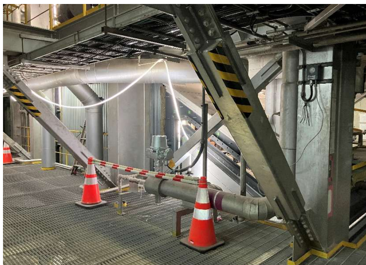
焼却炉ケーシング据付後
